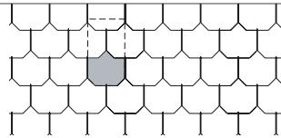
XL BASSA 720 x 400 mm Fachweite | Pureau 300 mm
