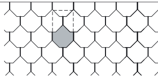
XL VIVA 720 x 400 mm Fachweite | Pureau 300 mm
