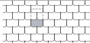
XM Ecken gestutzt | Angles rognés 600 x 400 mm Fachweite | Pureau 240 mm
