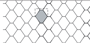
XM Waben | Losange 480 x 400 mm Fachweite | Pureau 180 mm
