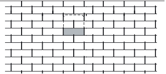
XM 400 x 400 mm Fachweite | Pureau 140 mm
