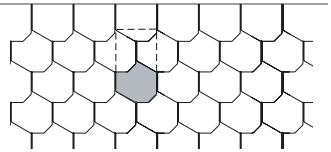
XL CREA 720 x 400 mm Fachweite | Pureau 300 mm
