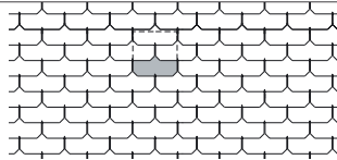
XM Ecken gestutzt | Angles rognés 400 x 400 mm Fachweite | Pureau 140 mm
