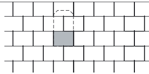
XL LINEA 720 x 400 mm Fachweite | Pureau 300 mm
