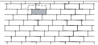
XL QUARDA 300 x 600 mm Fachweite | Pureau 180 mm
