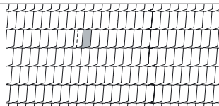
XS Steinschindeln | Bardeaux 300 x 200 mm Fachweite | Pureau 200 mm
